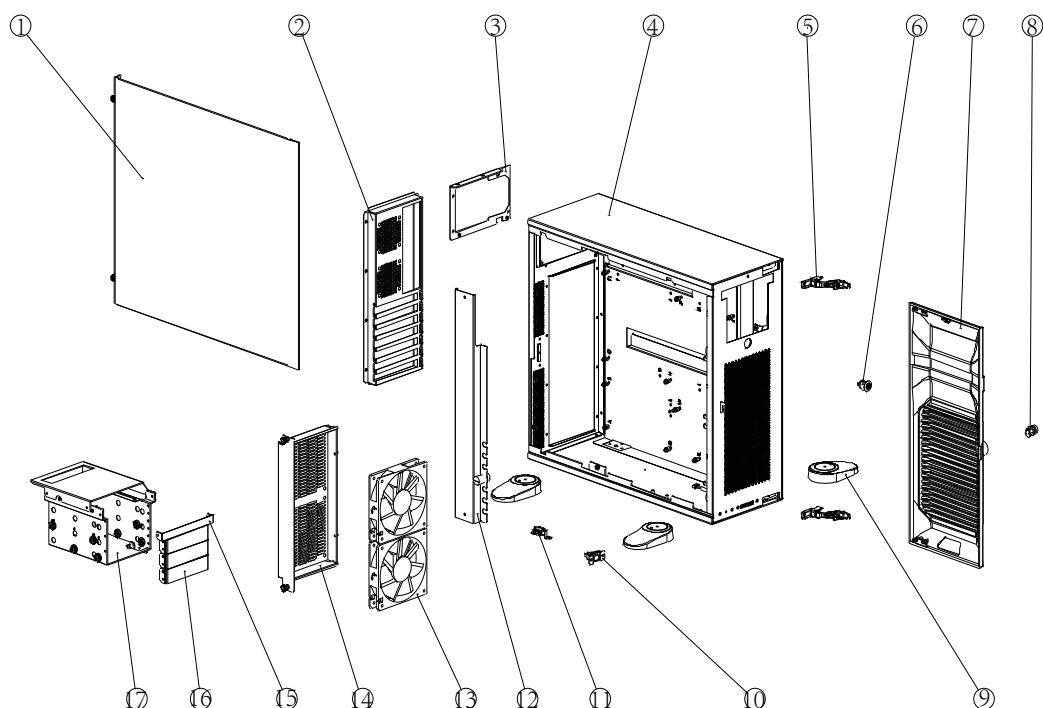
Figure A.1 Exploded Diagram & Parts List/ 分解图 & 部件列表 / 分解圖 & 零件表
