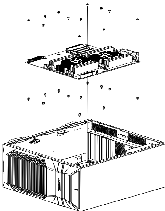
Figure 2.3 Fastening the stub copper and installing a motherboard/ 固定铜柱 & 安装主板 / 固定銅柱 & 安裝主板
